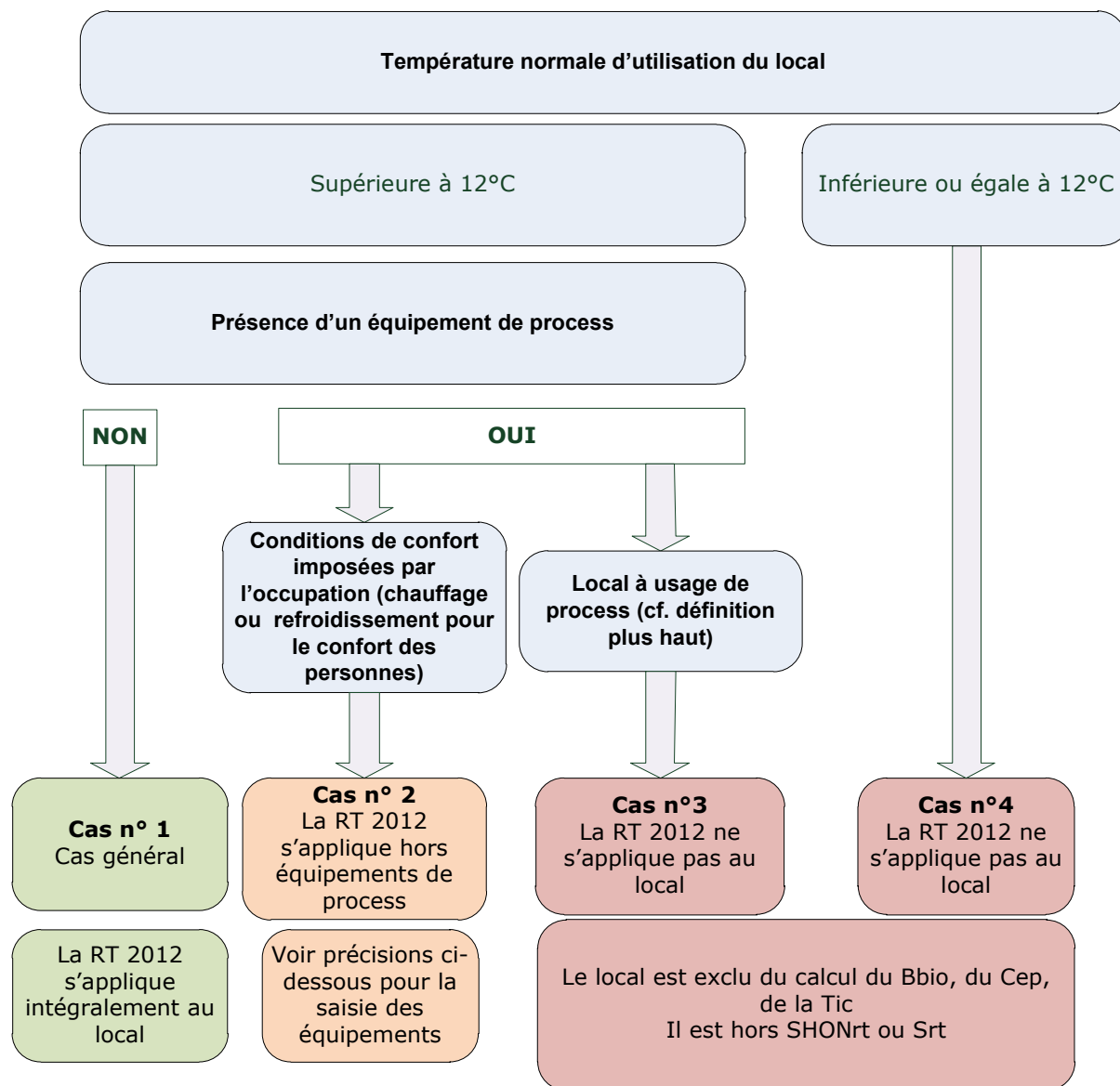
Figure 1 – schéma explicitant les limites d'application de la RT2012 pour les locaux à usage de process.
